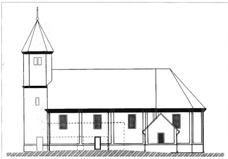
98. A templom déli homlokzata, építési periódusokkal
