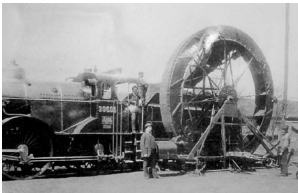
Schilhan-kerék a kanizsai állomáson
